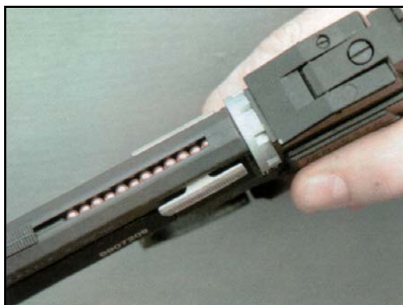
Рис. 3 Трубчатый магазин для стальных шариков ВВ расположен над стволом. При стрельбе шарик сначала попадает в барабан, и при его повороте подаётся на линию ствола.
